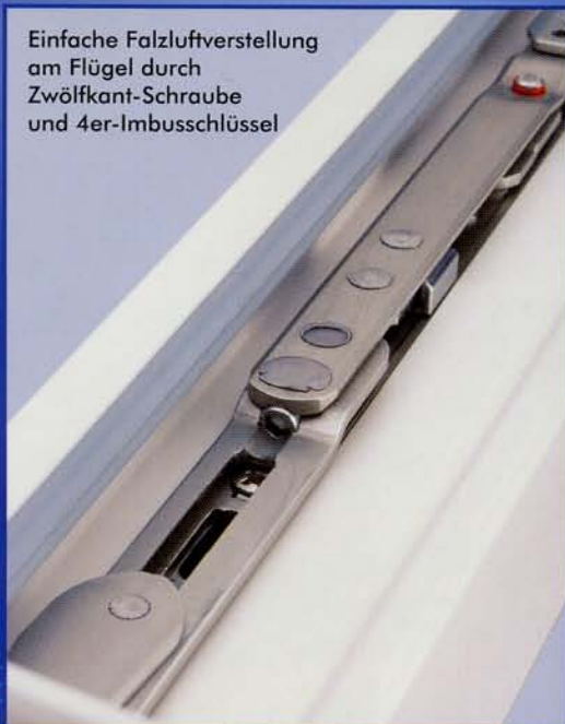
Weites Sichtfeld Roto NT Designo lässt sich bis zu 100° weit öffnen
