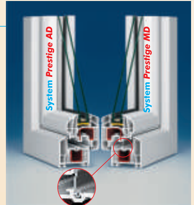
Das System MD verfügt über drei rundumlaufende Dichtungen. (Zwei bei System AD )
